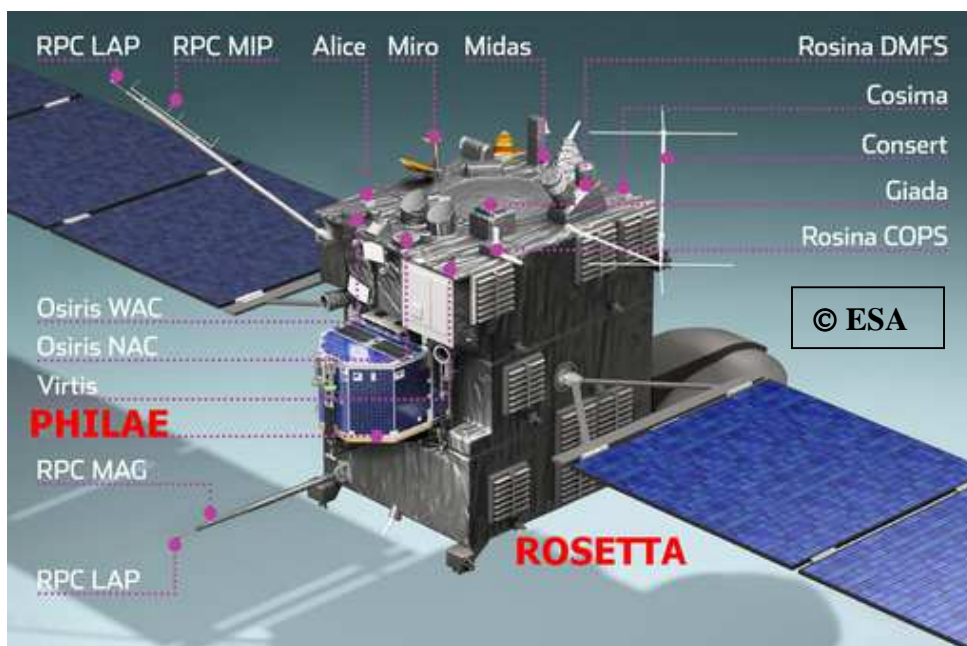
Rosetta et Philae : les différents instruments
