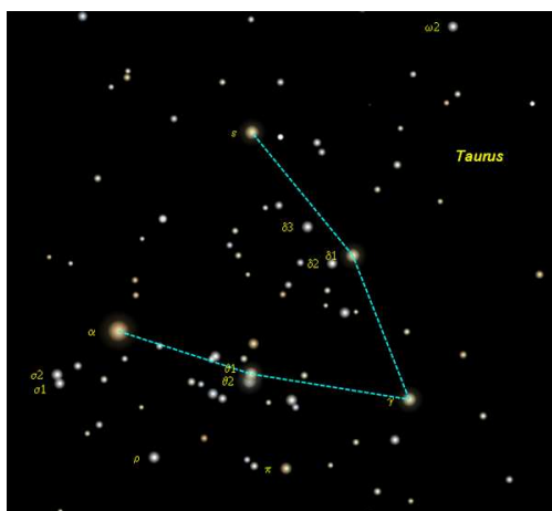
Le « V » de l'amas des Hyades.
