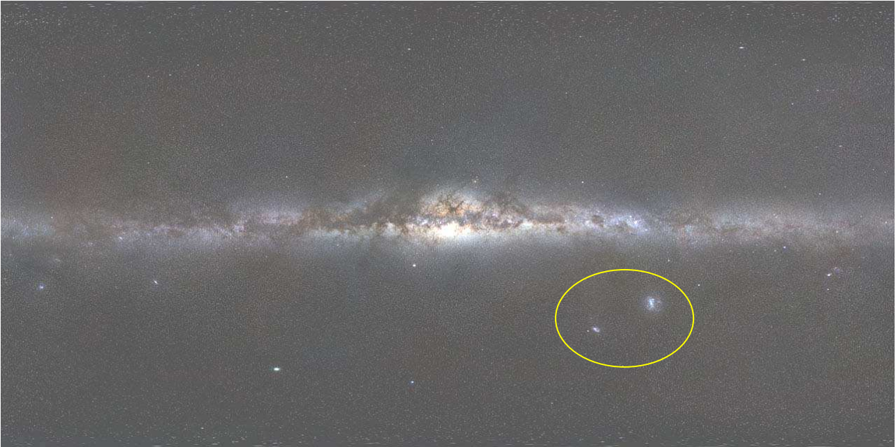
Image composite de notre Galaxie et des deux nuages de Magellan.
