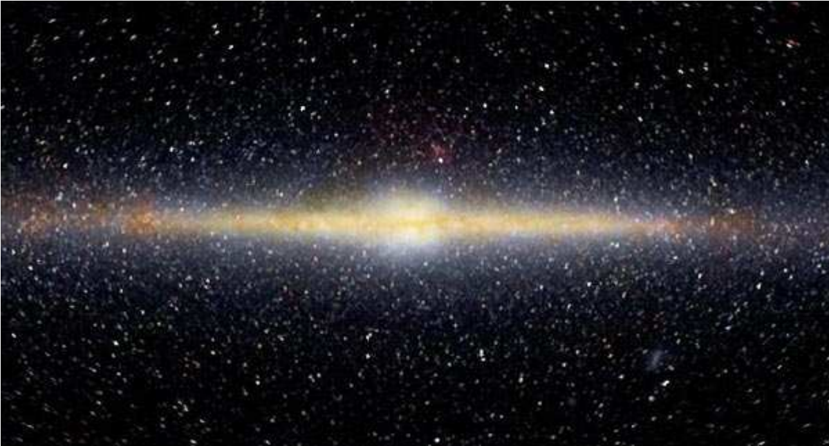
Représentation de notre Galaxie, la Voie Lactée.
